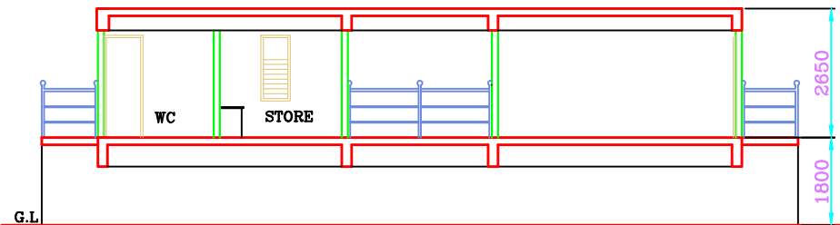
SECTION:B-B SCALE-1:100
