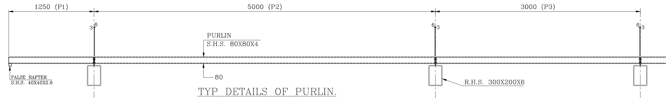
TYP DETAILS OF PURLIN.
