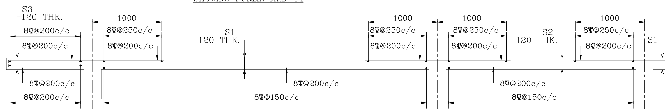
SECTION - A-A
