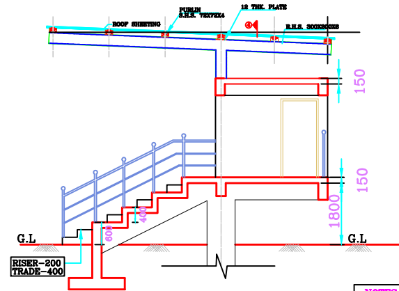
SECTION:A-A SCALE-1:100
