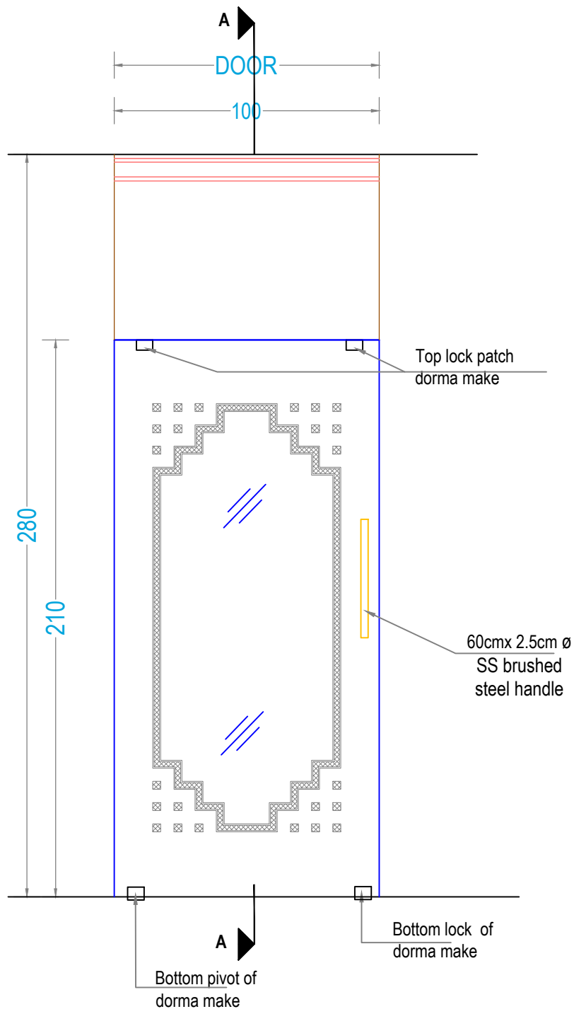
ELEVATION
