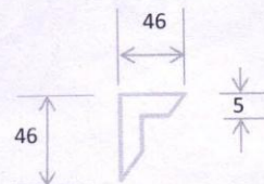
L- angle
